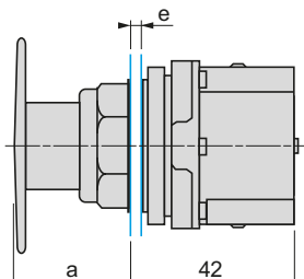
e: Stärke der Montageplatte: 1...6 mm
