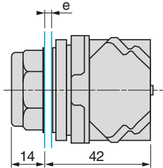
e: Stärke der Montageplatte: 1...6 mm
