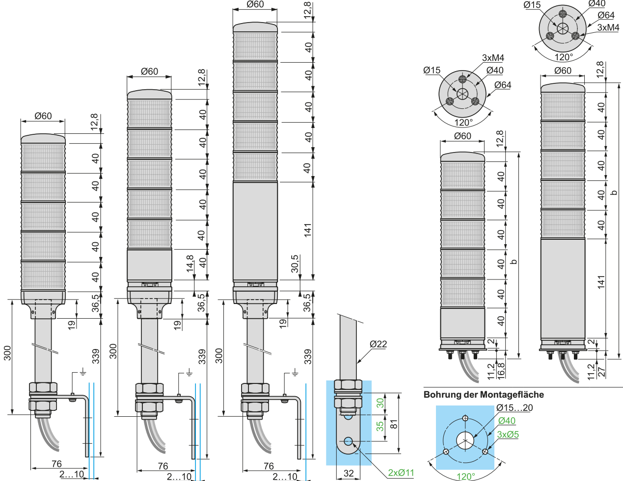
Höhe der vormontierten und verdrahteten Signalsäulen
