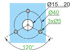
Bohrung der Montagefläche
