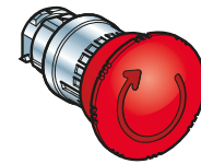
Drehentriegelung (EN/ISO 13850) ZB4BS8●4 siehe Seite 1/88
