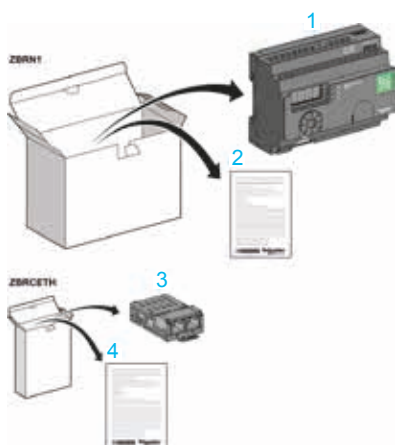
Abbildung A: ZBRN1: Der Harmony Hub in Standardausführung mit Kommunikationsmodul
