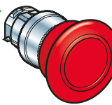
Zugentriegelung (EN/ISO 13850) ZB4BT84 siehe Seite 1/88
