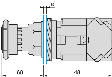
e: Stärke der Montageplatte: 1...6 mm
