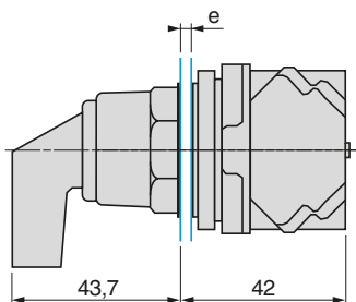
e: Stärke der Montageplatte: 1...6 mm
