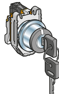
Schlüsselschalter XB4FG●● siehe Seite 1/111
