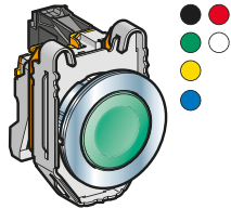
Flach, ohne Tastenbeschriftung XB4FA●1/FA42 siehe Seite 1/103
